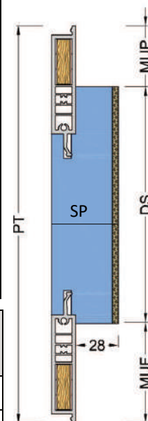
P30 CON PANNELLO ID 195
