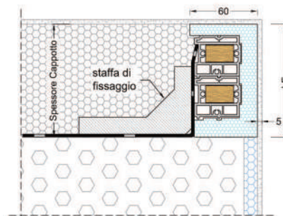
ID 1393 ESEMPIO STAFFA TIPO PESANTE
