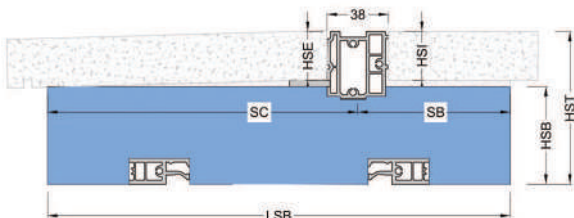
ESEMPIO DI INSTALLAZIONE A CENTRO MAZZETTA
