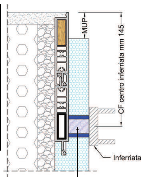
P30 CON ALLARGAMENTO
