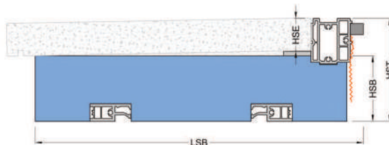
ESEMPIO DI INSTALLAZIONE A FILO MURO INTERNO
