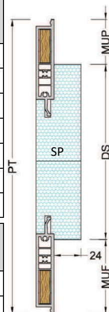
P30 CON PANNELLO ID 194
