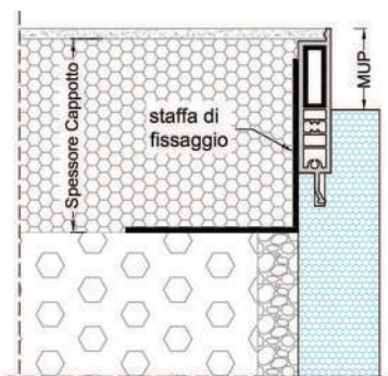
ID 1383 ESEMPIO STAFFA TIPO LEGGERO
