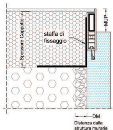
RINFORZO INTERNO SU P30
